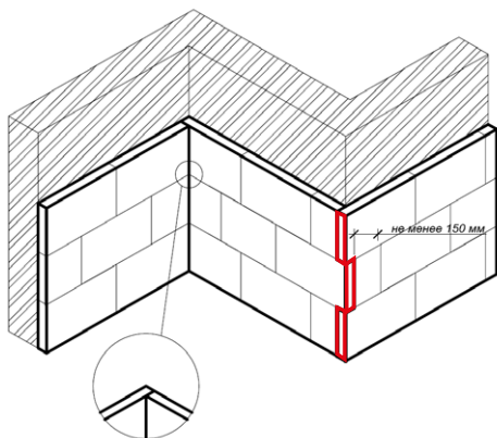
Рис. 9. Схема перевязки плит на внутренних и наружных углах здания
