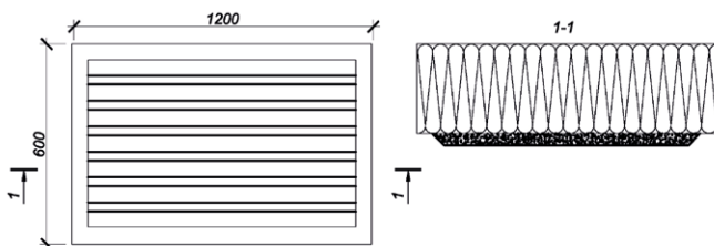
Рис. 5. Схема сплошного нанесения клея на плиту
