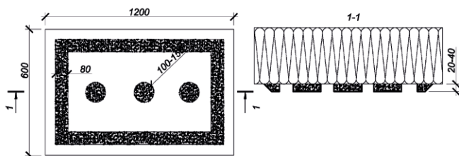
Рис. 7. Схема точечного (контурно-маячкового) нанесения клея на плиту
