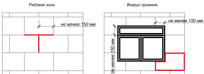
Рис. 11. Схема установки плит на плоскости фасада и вокруг проемов
