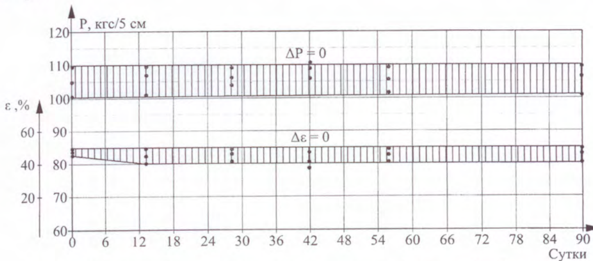
Рис. 2. Изменение прочности (1) и относительного удлинения (2) образцов рулонного материала "Техноэласт АЛЬФА" при воздействии 15-% раствора H 2 SO 4
