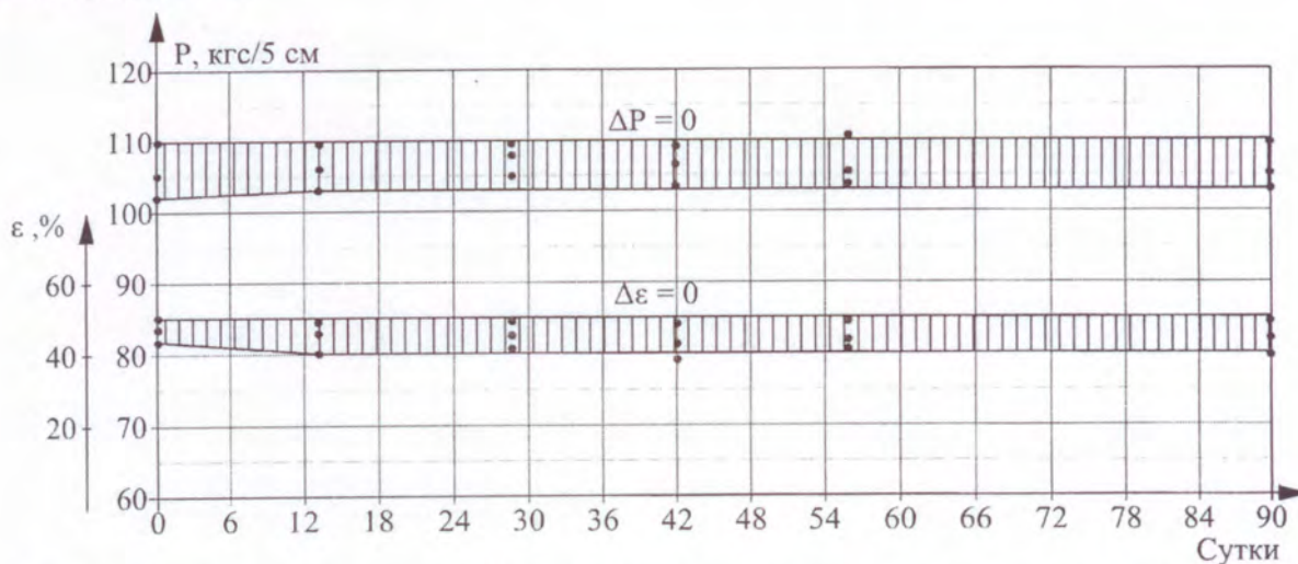
Рис. 1. Изменение прочности (1) и относительного удлинения (2) образцов рулонного материала "Техноэласт АЛЬФА" при воздействии 15-% раствора NaOH
