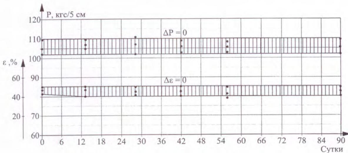
Рис. 3. Изменение прочности (1) и относительного удлинения (2) образцов материала "Техноэласт АЛЬФА" при воздействии насыщенного раствора NaCl
